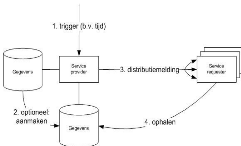
Figuur B2. Use case '(multi-) distributie'
