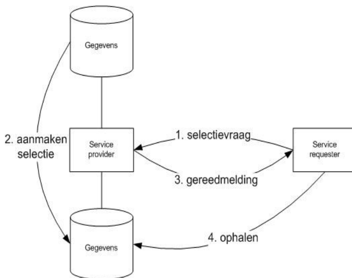
Figuur B3. Use case 'Selectie'
