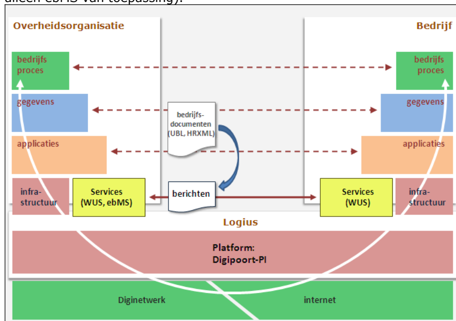
Figuur 2: Digiport koppelvlak t.b.v. DigiInkoop/E-Facturieren
